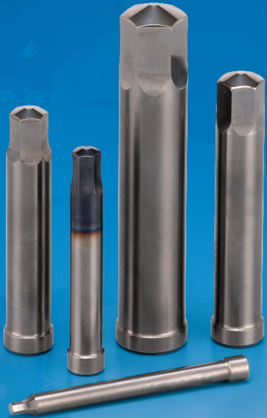
Carbide Punches
